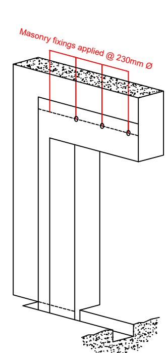
R.C. LINTEL
