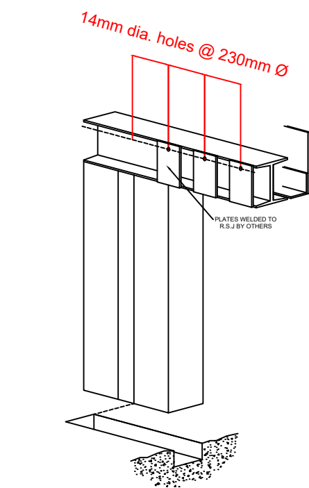
R.C. LINTEL
