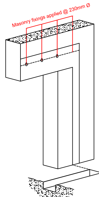
R.C. LINTEL
